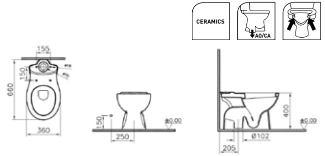
STAANDE WC - 660 MM - S-UITGANG 20,5 CM CUVETTE - 660 MM - S 20,5 CM WC BODENSTEHEND - 660 MM - ABGANG INNEN SENKRECHT 20,5 CM
