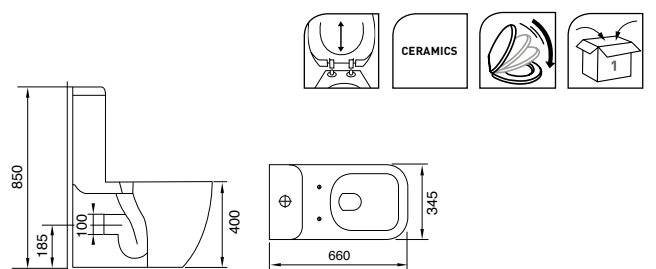
PACK STAANDE WC UITGANG H PACK WC À POSER SORTIE H PACK STAND-WC H ABGANG
