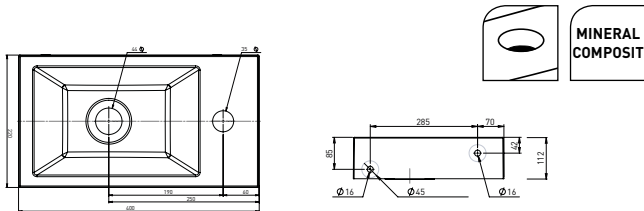
HANDENWASSER RECHTS 400 X 220 MM LAVE-MAINS DROITE 400 X 220 MM HANDWASCHBECKEN RECHTS 400 X 220 MM
