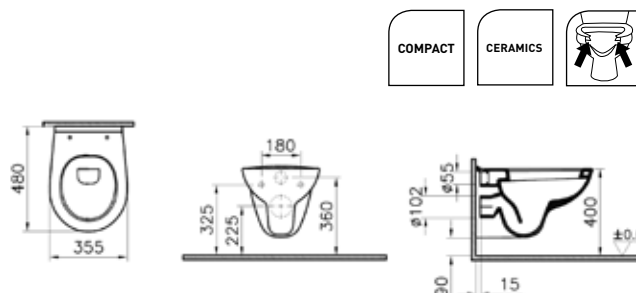
HANGTOILET - VERKORT - 480 MM WC SUSPENDU - COURT - 480 MM WAND-WC - KURZ - 480 MM
