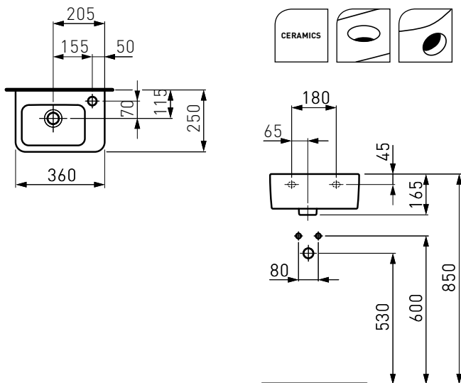
HANDENWASSER KRAANGAT RECHTS 360 X 250 MM LAVE-MAINS AVEC TROU ROBINET DROITE 360 X 250 MM HANDWASCHBECKEN MIT HAHNLOCH RECHTS 360 X 250 MM
