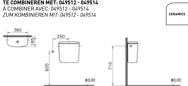
JACHTBAK MET MECHANISME 3/6L RÉSERVOIR AVEC MÉCANISME 3/6L SPÜLKASTEN MIT GARNITUR 3/6L
