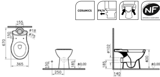
STAANDE WC - 670 MM - H-UITGANG 18,5 CM CUVETTE - 670 MM - H 18,5 CM WC BODENSTEHEND - 670 MM - ABGANG WAAGERECHT 18,5 CM
