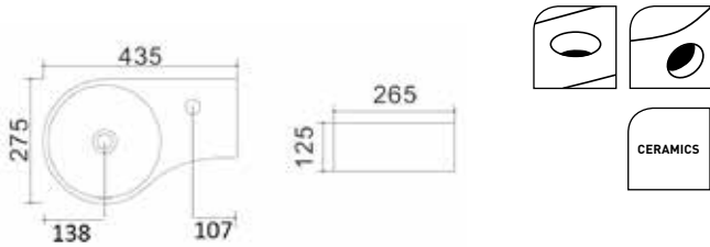
HANDENWASSER RECHTS 435 X 275 MM LAVE-MAINS DROITE 435 X 275 MM HANDWASCHBECKEN RECHTS 435 X 275 MM
