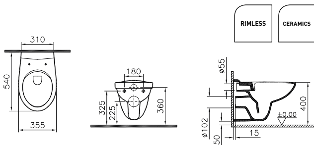
HANGWC RIMLESS - 540 MM CUVETTE SUSPENDUE - RIMLESS - 540 MM WAND-WC - RIMLESS - 540 MM
