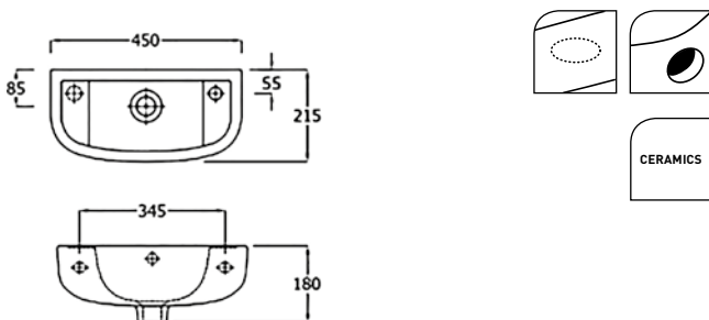
HANDENWASSER 450 X 215 MM LAVE-MAINS 450 X 215 MM HANDWASCHBECKEN 450 X 215 MM
