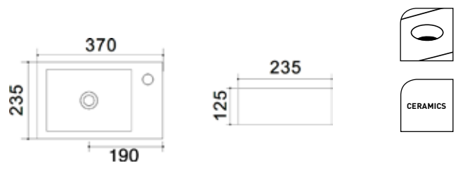
HANDENWASSER RECHTS 370 X 235 MM LAVE-MAINS DROITE 370 X 235 MM HANDWASCHBECKEN RECHTS 370 X 235 MM
