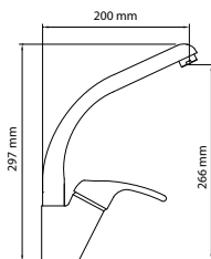
KEUKENMENGKRAAN EENGREEPS MET HOGE BEK MITIGEUR CUISINE AVEC BEC HAUT EINHAND-SPÜLTISCHBATTERIE
